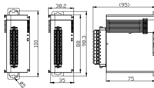
AS02LC-A / AS04AD-A / AS04DA-A / S04TC-A / AS04RTD-A / AS06XA-A / AS08AD-B / AS08AD-C / AS06RTD-A / AS08TC-A
